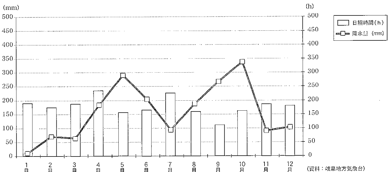
●月別降水量と日照時間（平成16年）
