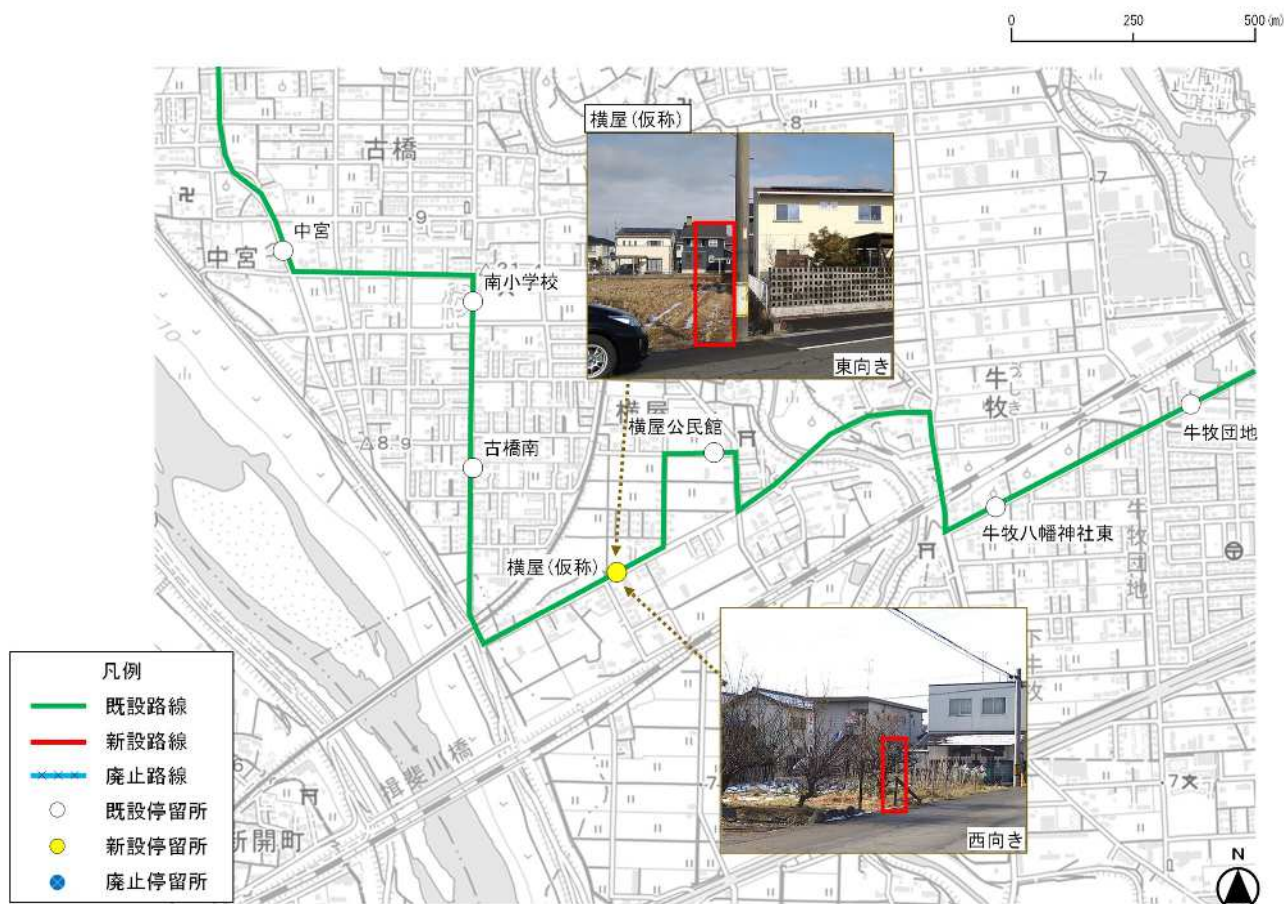
横屋(仮称)バス停位置図
