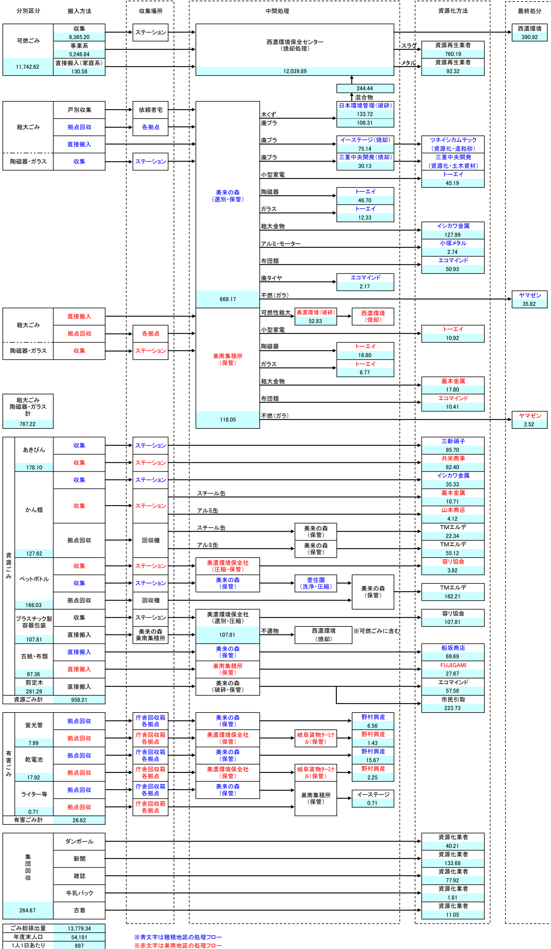
ごみ処理フロー（瑞穂市全体・平成29年度）
