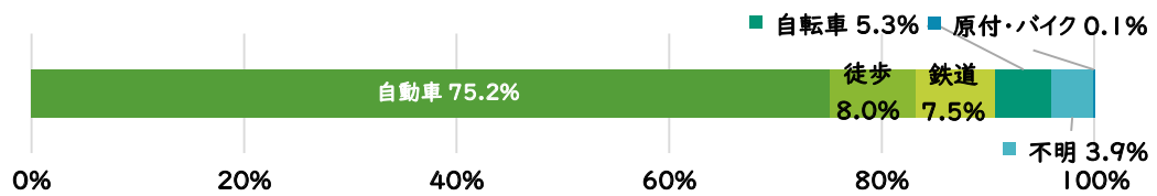
図3-18 手段分担率
