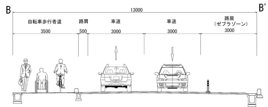
断面図 新設道路 (B-B')
