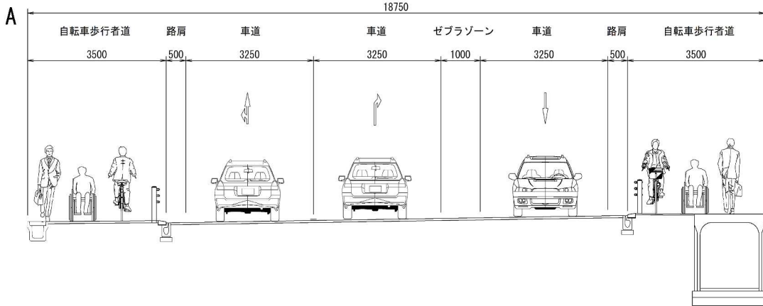
断面図 市道4-1009号線 (A-A')
