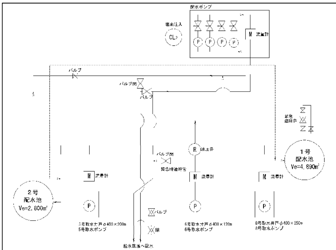
図 2.6 別府水源地施設の概要
