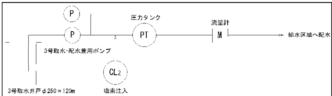
図 2.4 牛牧水源地施設の概要
