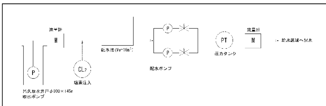
図 2.8 呂久水源地施設の概要
