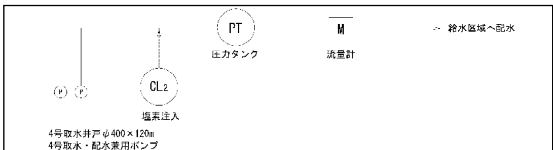
図 2.5 本田水源地施設の概要
