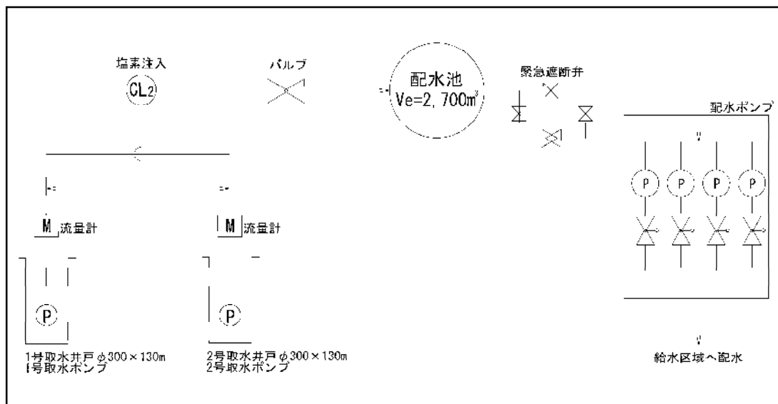
図 2.3 宮田水源地施設の概要
