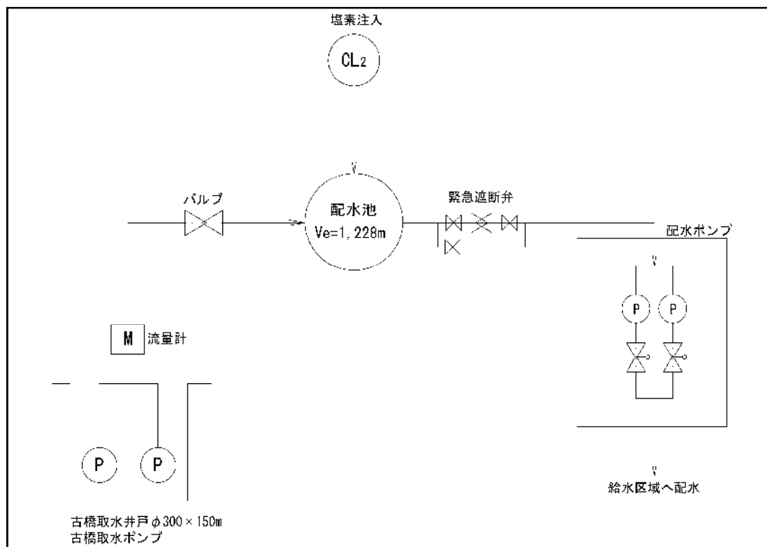
図 2.9 古橋水源地施設の概要
